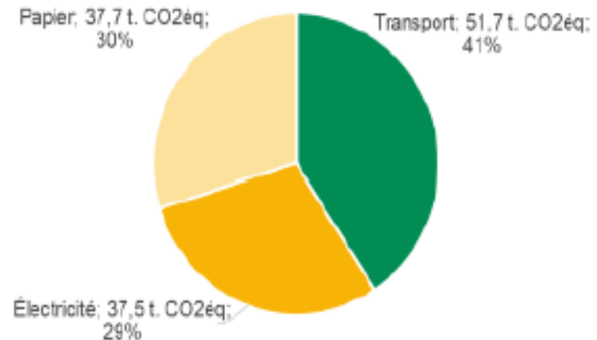
Émissions de gaz à effet de serre du CFE Tunisie 2018
